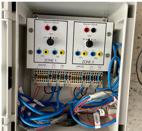
Aangesloten monitoringbox
